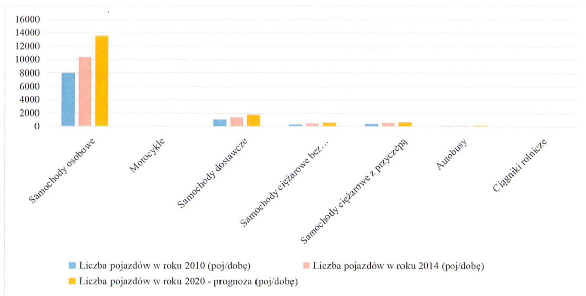
Rysunek 8 Średnio dobowy ruch na DW385
