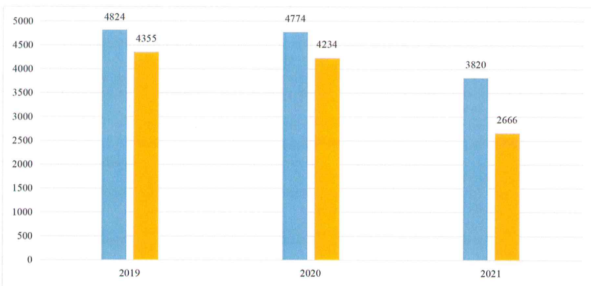
Rysunek 24 Ilość zebranych odpadów komunalnych na terenie gminy Ziębice w latach 2019-2021
