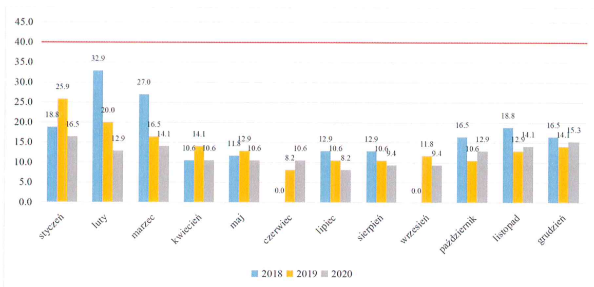
Rysunek 4 Średnie stężenie dwutlenku azotu na stacji w Żąbkowicach Śląskich w latach 2018 – 2020 ( \mu\text{g}/\text{m}^3 )
