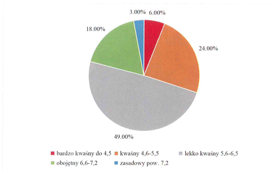
Rysunek 18 Odczyn gleb użytkowanych rolniczo w powiecie ząbkowickim w latach 2012-2015 Źródło: OSCHR Wrocław
